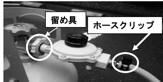
図2 圧力調整器 (ガスボンベ接続)
