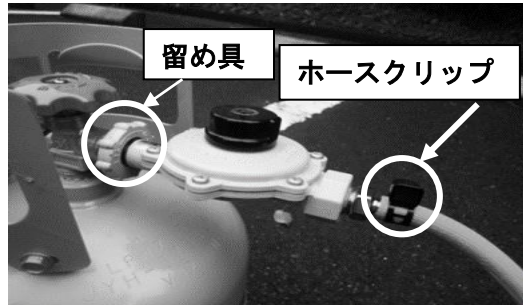
図3 圧力調整器 (ガスボンベ接続)
